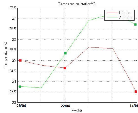
Fig. 6. Evolución de temperature in silo A05
