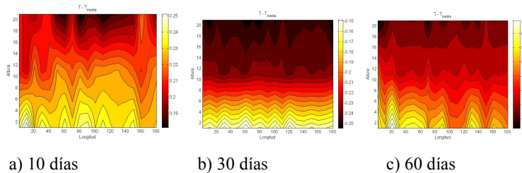
Fig. 7. Termografía NIR para silo A05
