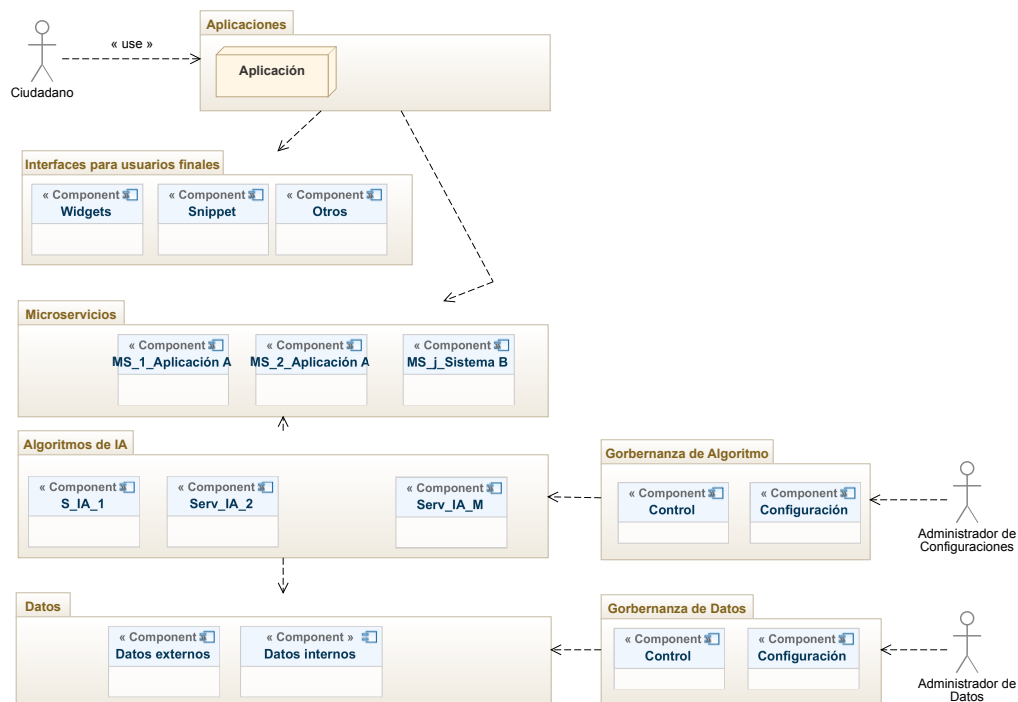
Fig. 1. Arquitectura conceptual
